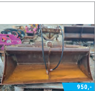
Grabenräumlöffel KL1.2 GRS170 SI11 für Bagger 5,5-9 t, SI11, Inhalt 0,43 m³, Breite 1700 mm, Gewicht 520 kg leicht gebraucht BJ 2014, SNr. 14/26258
