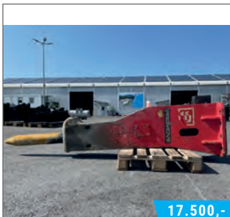
Hydraulikhämmer PROMOVE XP1700 für Bagger 19-28 t, Gewicht 1.700 kg, mit Meißel und Schmiersystem, gebraucht, BJ 2018, SNr. PRO.3218019
